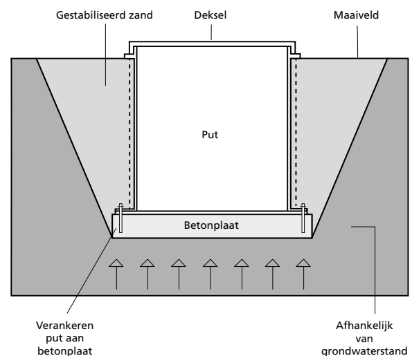
Inbouwwijze technieputten
