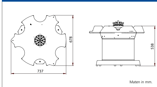
Maatschets AT 15 F
