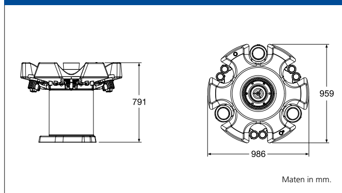
Maatschets AT 30 F en 35 F
