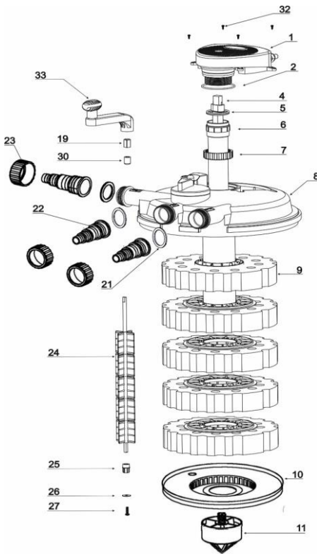
B VarioPress 7000/14000
